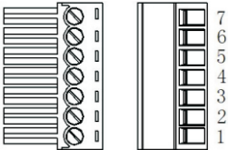
图 10-2 外端子插头示意图
